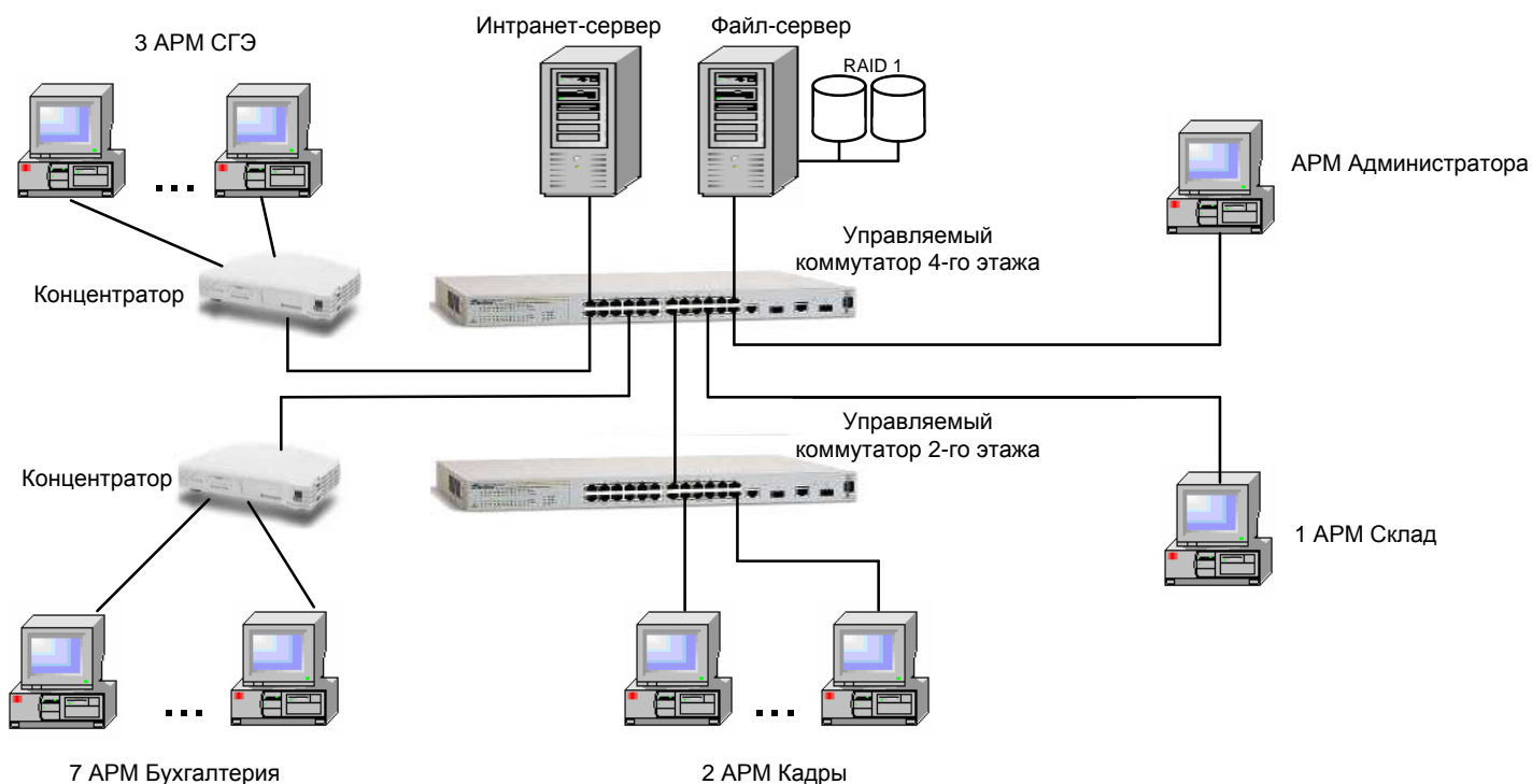
Общая схема АСЭМ «Клен».
